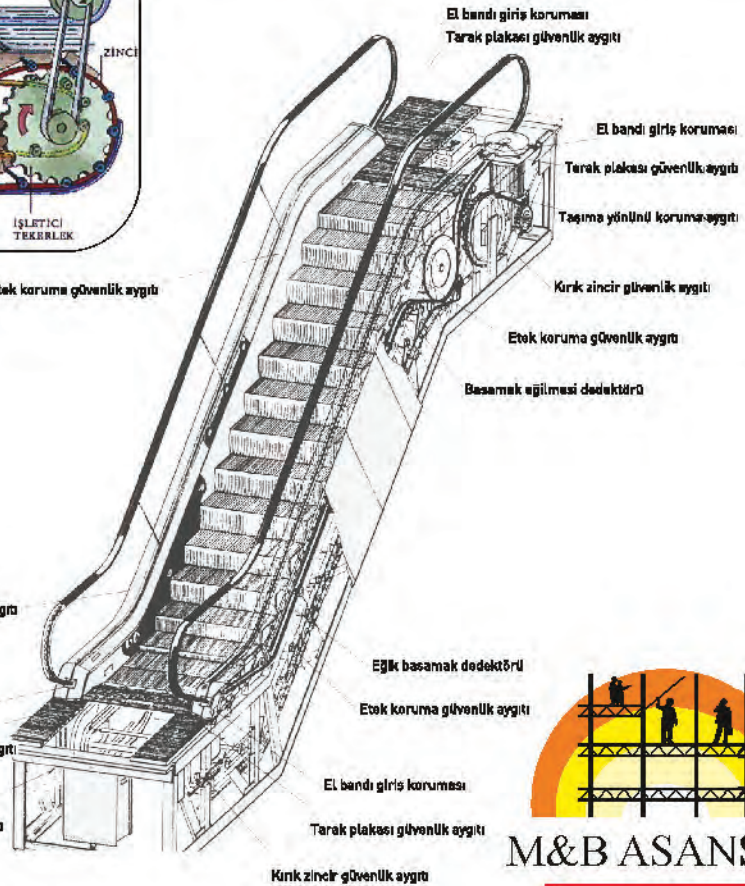
Kırık zincir güvenlik aygıtı
